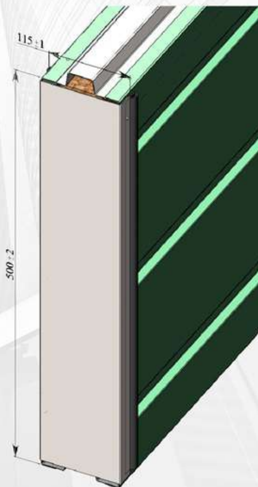
Габаритные размеры панели
